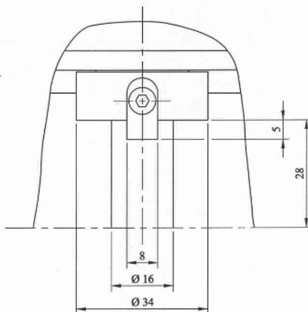
Ansicht A
