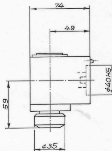
Spannzange EX, ESX 20 Spann.bereich : 1 ÷ 13
