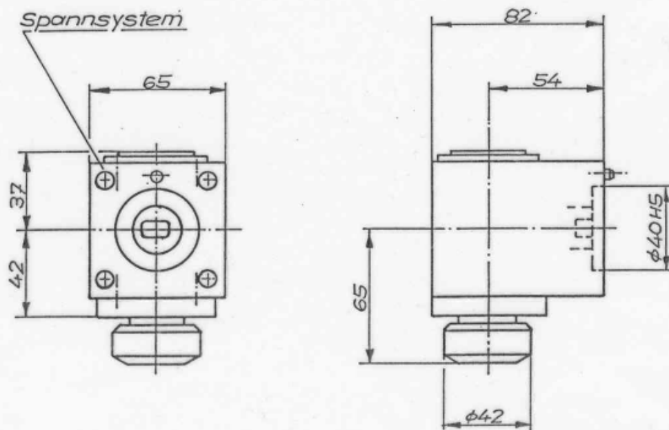
Spannzange EX, ESX 25 Spann.bereich : 1 ÷ 16
