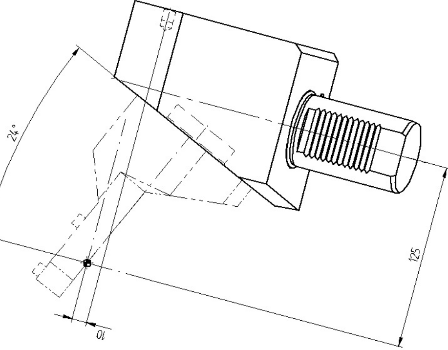
Ansicht A
