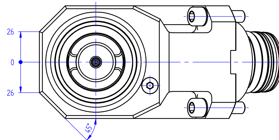
Ansicht A view A vue A
