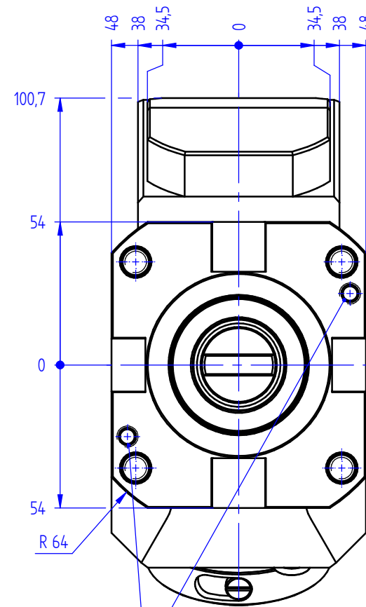
Ansicht A view A vue A
