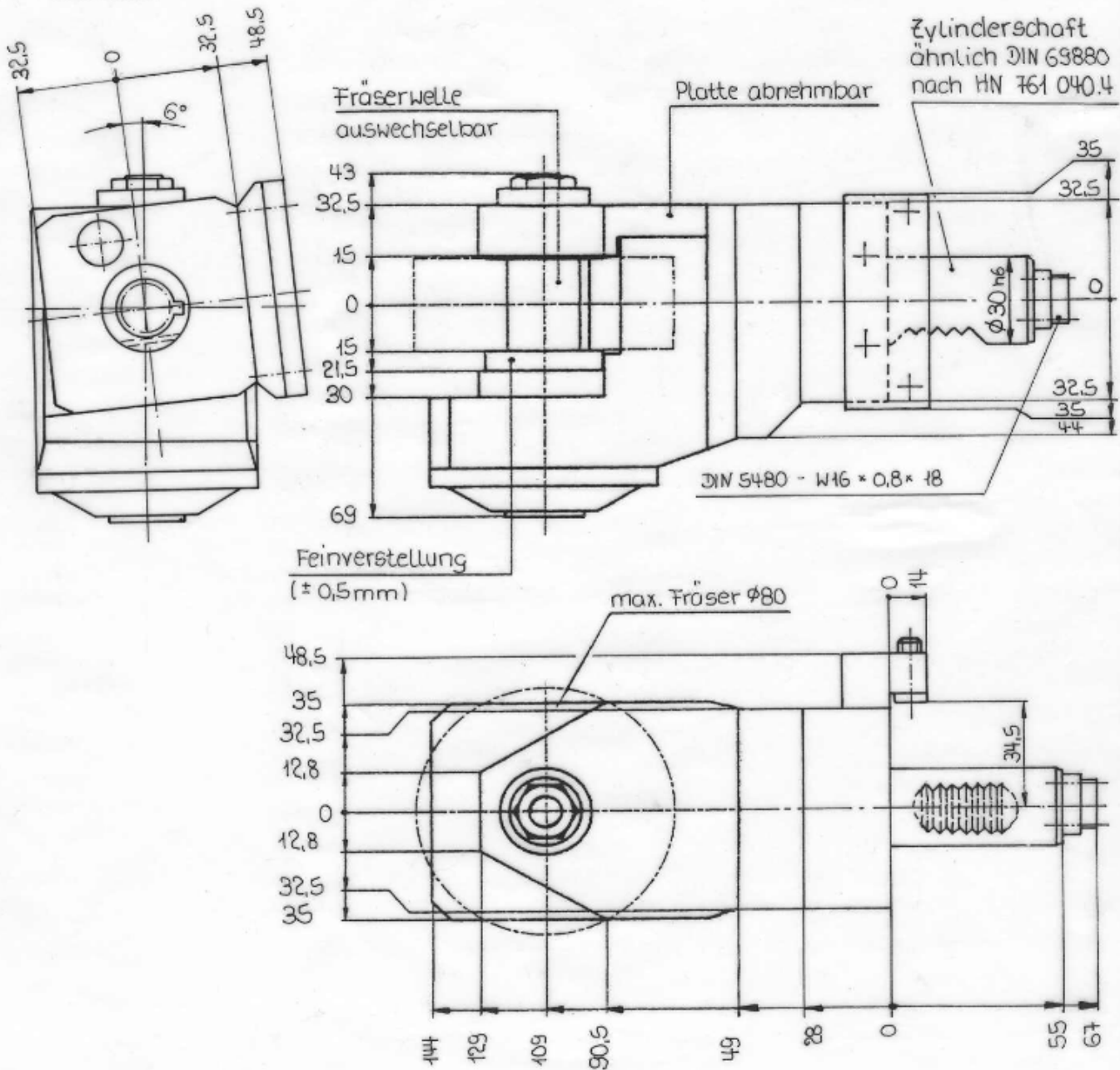
Fräserwelle kpl.
