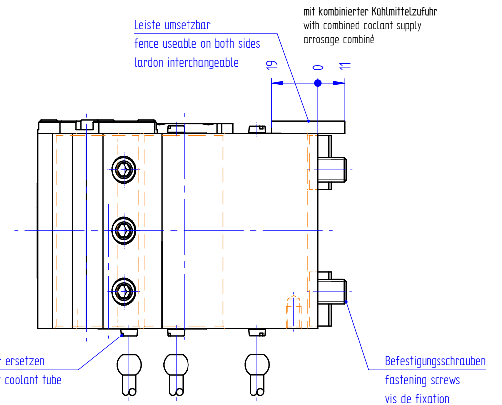
Ansicht A view A vue A
