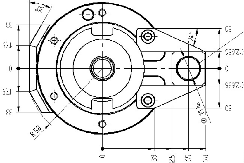
Schwenkkopf 7 049 45 004 Milling and drilling head, swivelling 7 049 45 004 Tête pivotante 7 049 45 004
