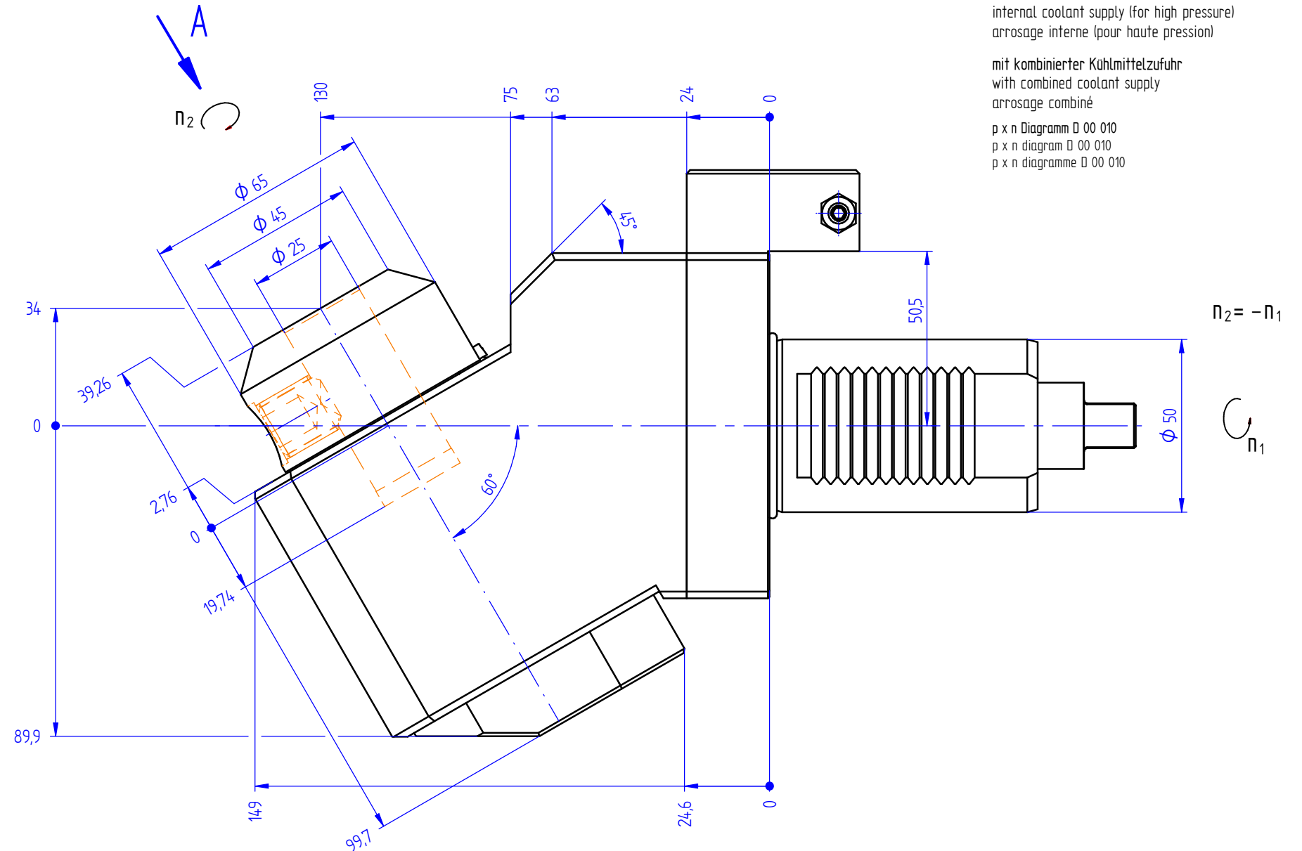
Ansicht A
