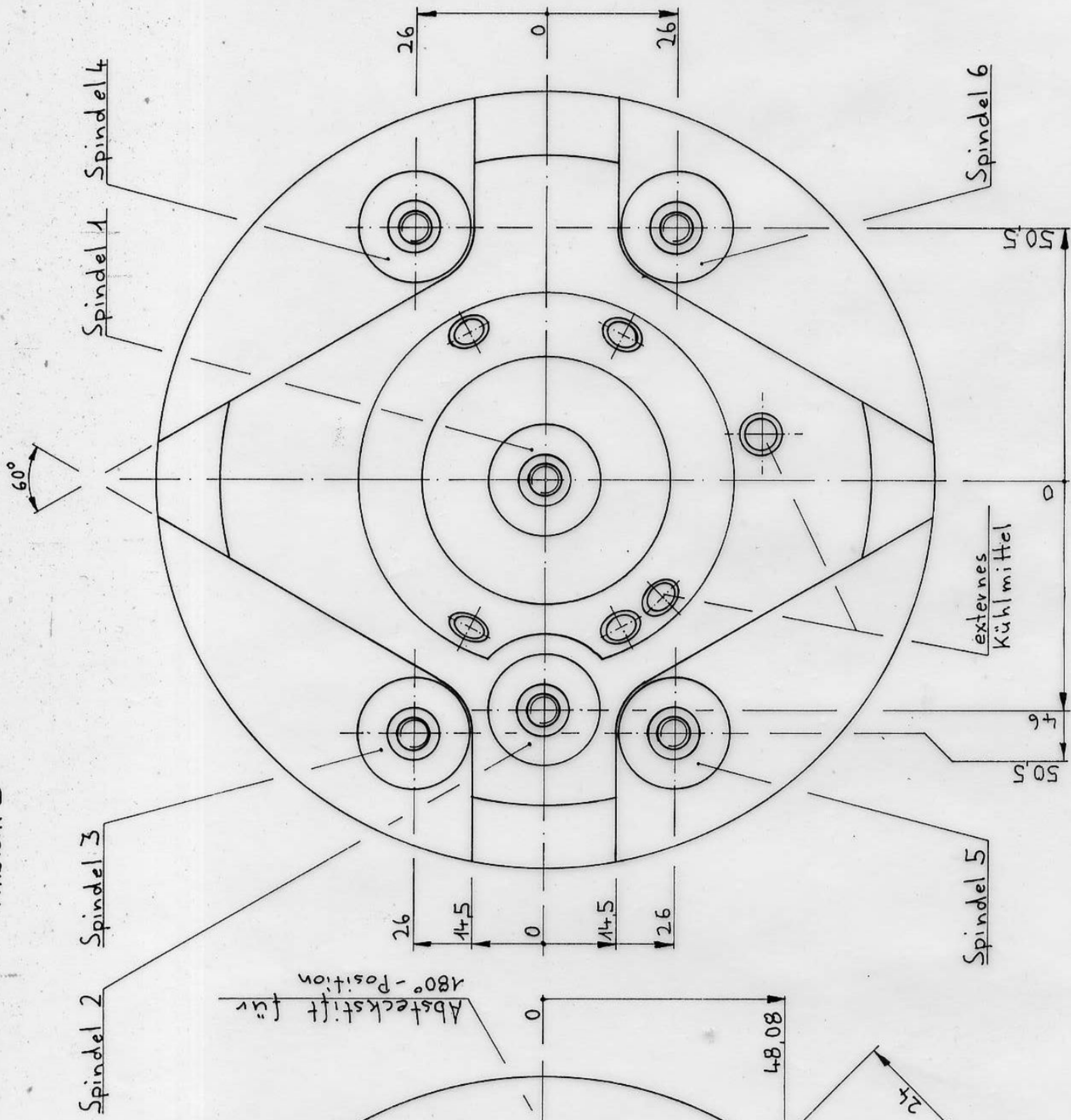
Ansicht B
