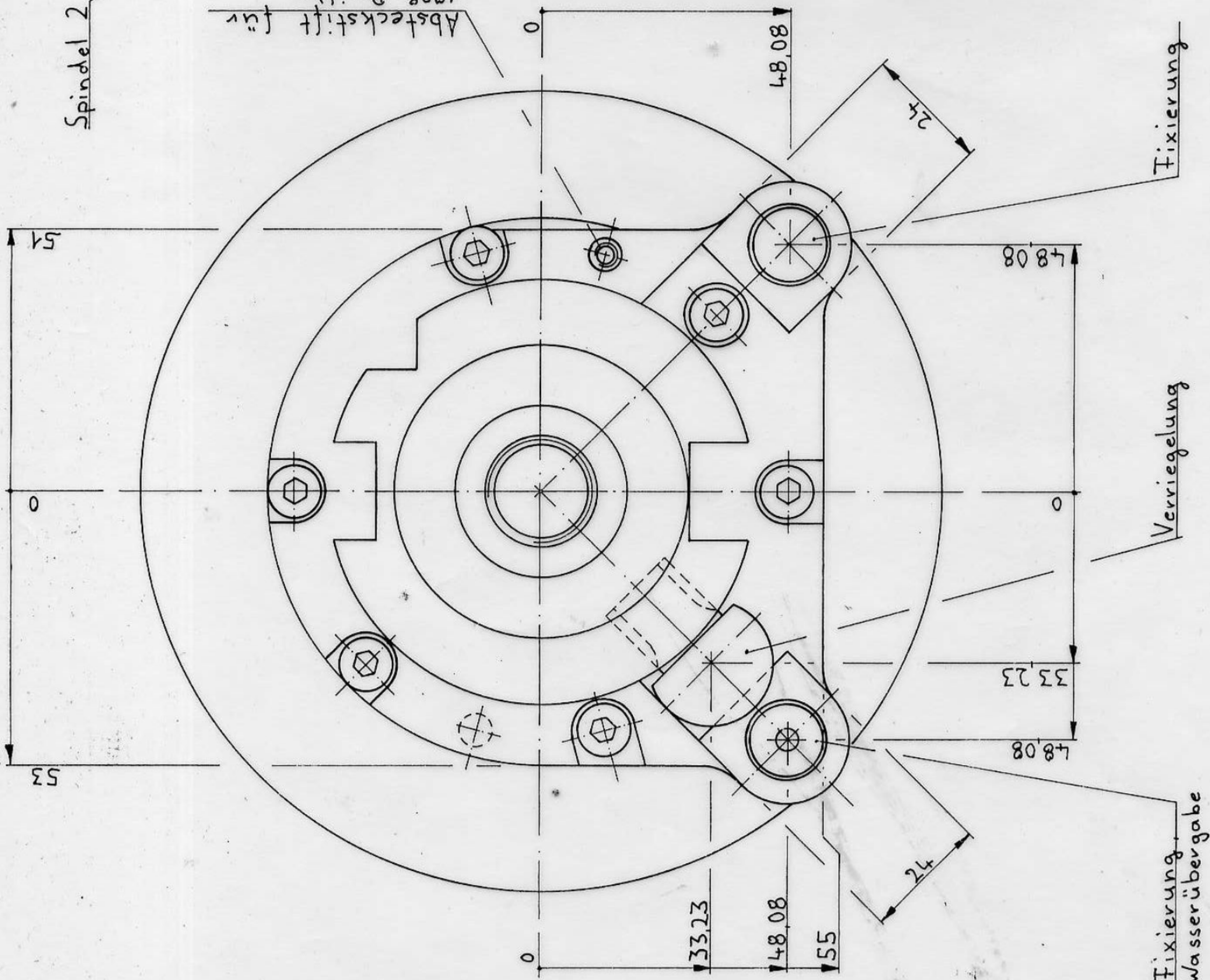
Ansicht A
